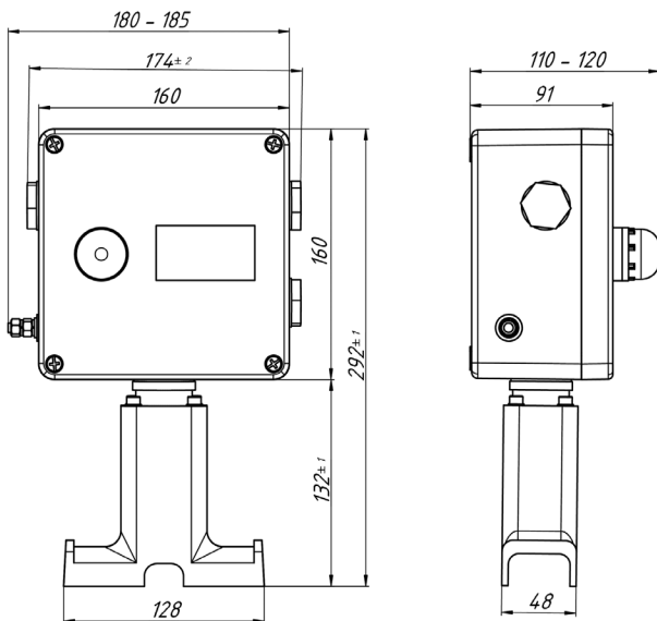
Габаритные размеры
