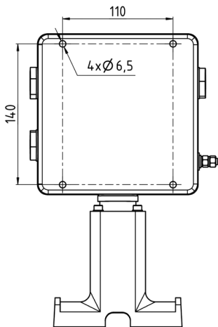
Установочные размеры
